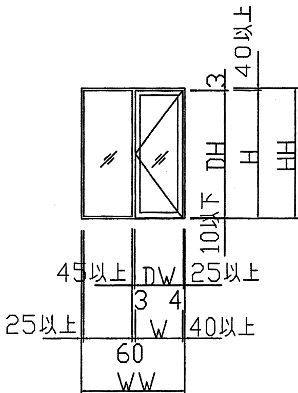
図4 片開き戸の形式
