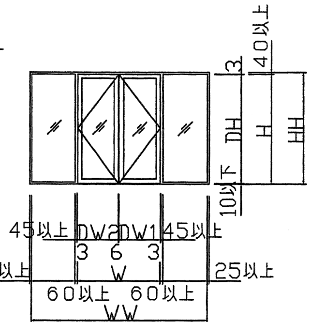
②両袖付き、欄間無し
