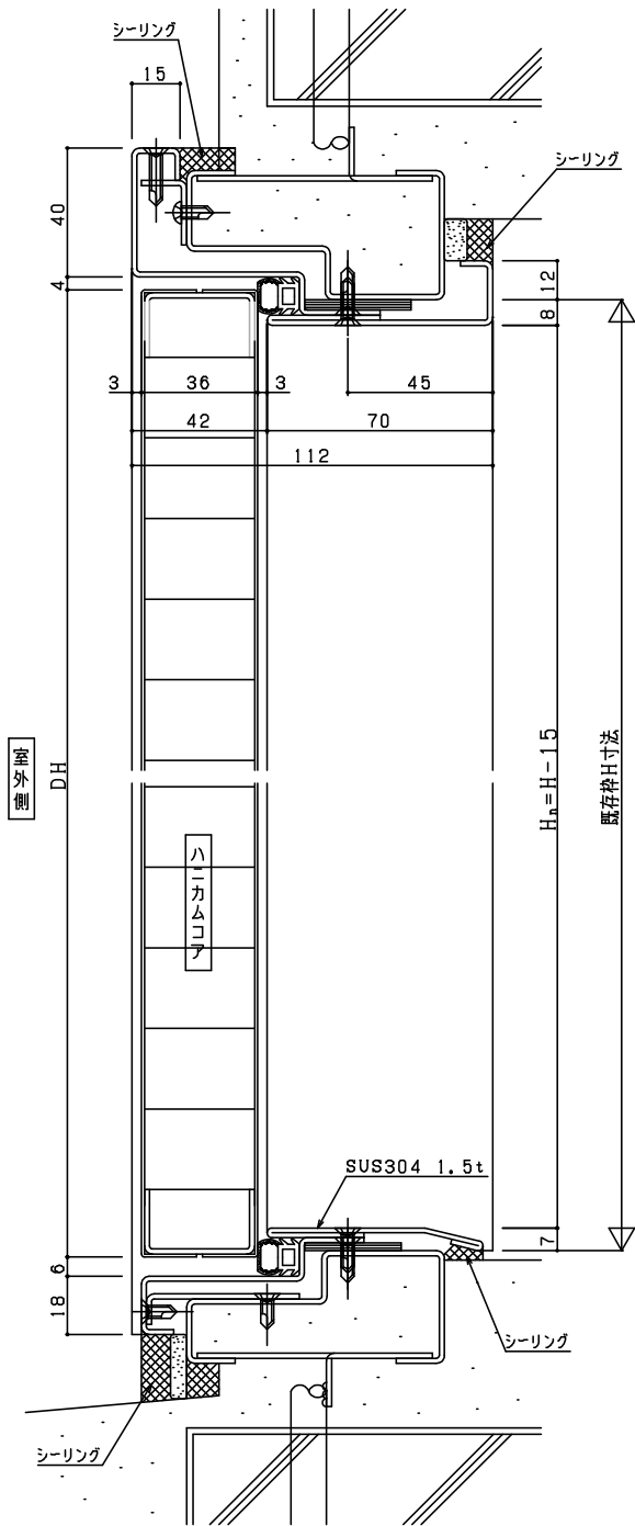
縦断面図
