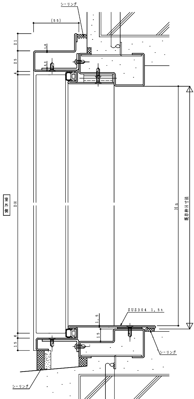
縦断面図
