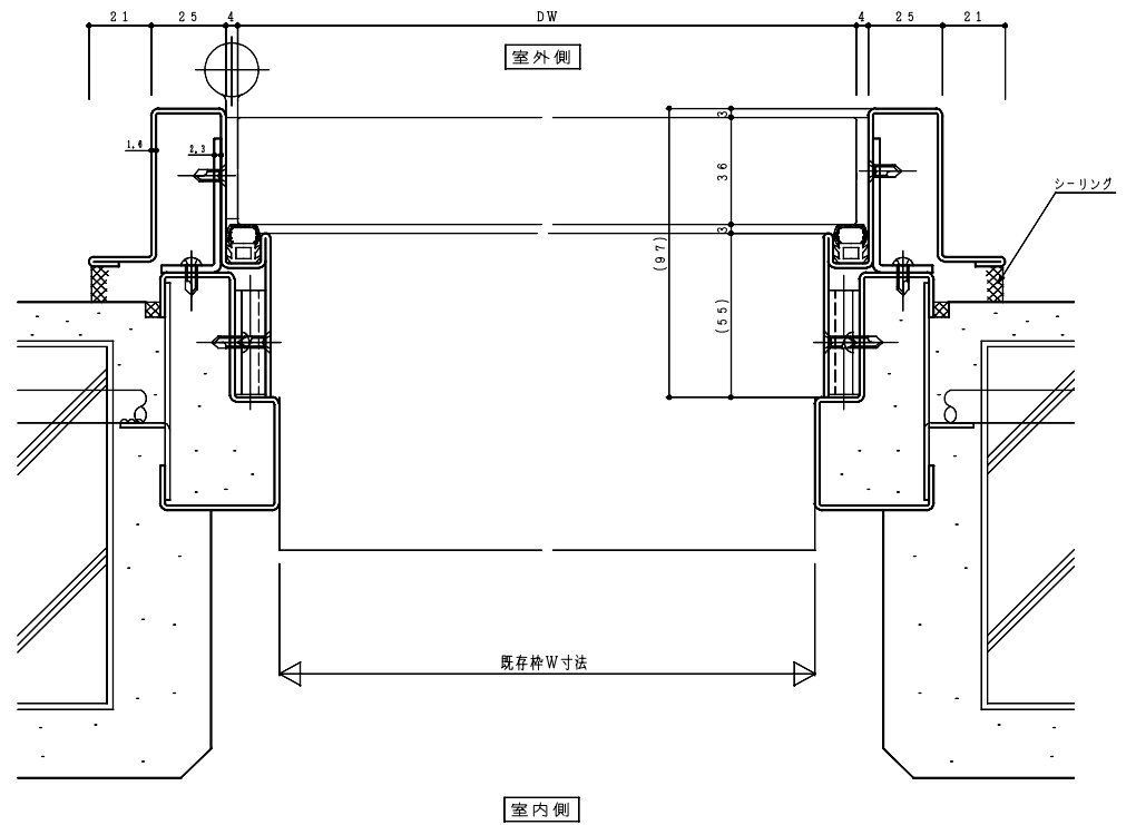
横断面図
